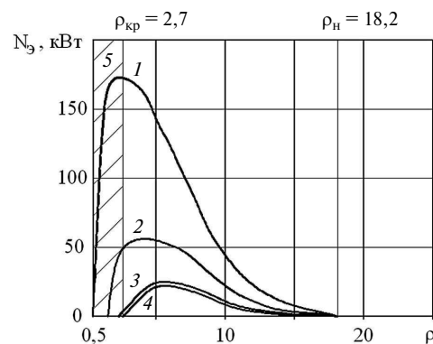
Рис. 2. Мощность, рассеиваемая на буксующем элементе управления в трансмиссии гусеничной машины при повороте с относительным радиусом меньше \rho_H .
