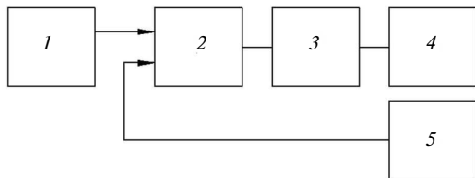
Рис. 3. Структура следящей системы управления поворотом, использующей широтно-импульсную модуляцию давления: 1 — датчик; 2 — дифференциальный усилитель; 3 — широтно-импульсный модулятор; 4 — объект управления (фрикционный элемент управления); 5 — датчик обратной связи
