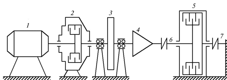
Рис. 4. Кинематическая схема стенда для испытаний ФЭУ и СУП: 1 — электродвигатель; 2 — фрикционная муфта для нагружения стенда; 3 — маховик; 4 — понижающий редуктор; 5 — испытываемый ФЭУ; 6 — входной вал муфты 5; 7 — тензометрический вал
