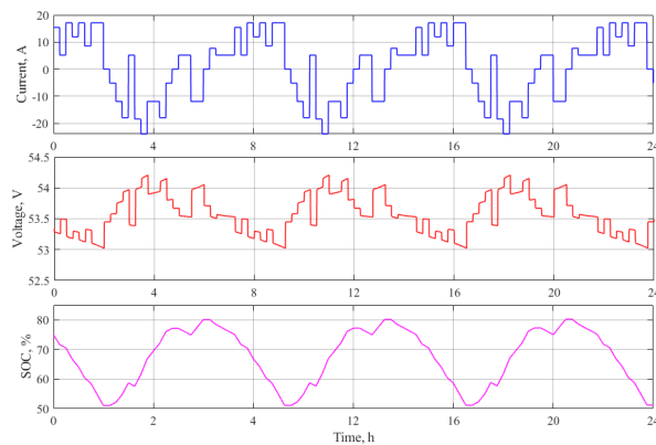
Рис. 5. Результаты моделирования режимов батареи ESS-5120 при эксплуатации по профилю автономных энергетических систем на основе ВИЭ
