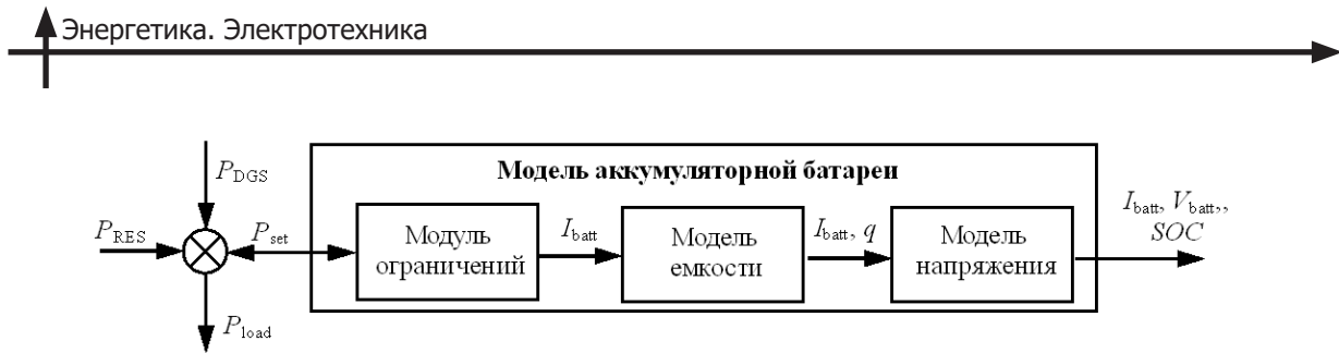
Рис. 3. Функциональная схема модели аккумуляторной батареи
