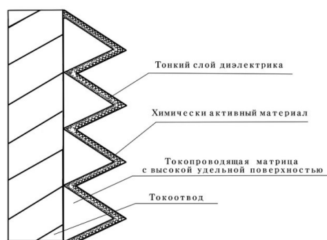
Рис. 1. Модель перспективного электродного материала гибридного конденсатора
