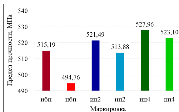
Рис. 5. Значения предела прочности для экспериментальных образцов
