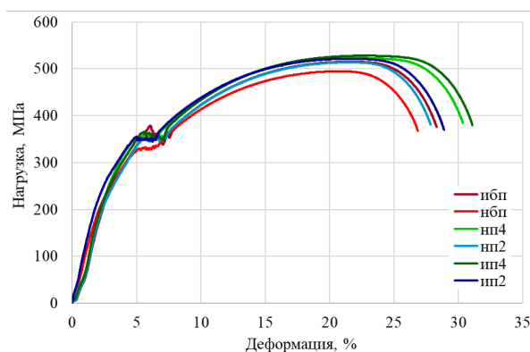
Рис. 4. Диаграммы деформации для испытанных экспериментальных образцов
