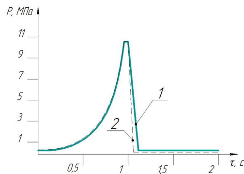
Рис. 3. График изменения мгновенного давления в рабочей камере:
