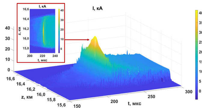
Рис. 3. Высотно-временной профиль тока сильнотоочного разряда.
