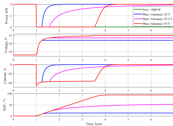
Рис. 6. Изменения параметров батареи ESS-5120 в режиме заряда при разных уставках на величину максимального напряжения заряда
