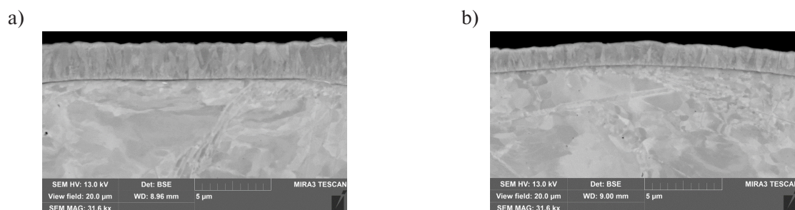
Рис. 2. Микроструктура барьерного покрытия экспериментального образца со средней толщиной \sim 2 мкм без наводороживания (a) и после наводороживания (b)
