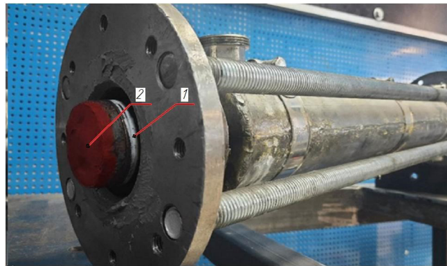
Рис. 2. Вид поршня с резиновым диском: 1 – поршень, 2 – резиновый диск
