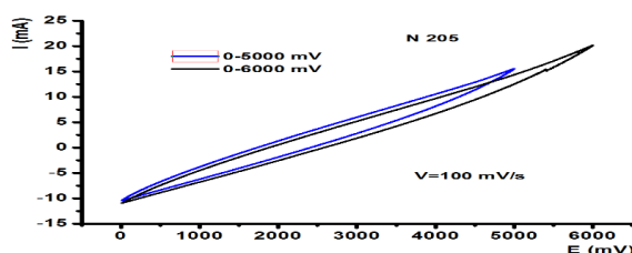
Рис. 6. Циклическая вольтамперограмма конденсатора с модифицированными титаном электродами
