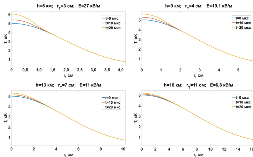
Рис. 10. Результаты численного решения уравнения теплопроводности на различных высотах, подтверждающие ухудшение условий формирования и поддержания горячего лидерного канала с ростом высоты над землей. На всех высотах напряженность электрического поля в канале составляет 10% от порога поддержания роста положительных стримеров, равного 500 кВ/(м·атм)
