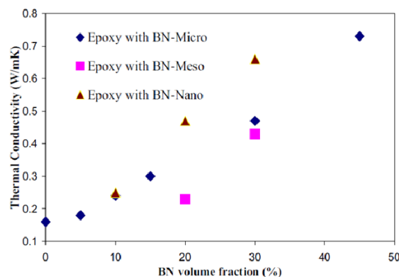
Рис. 2. Теплопроводность эпоксидных композитов с нано / мезо / икпоразмерными частицами BN
