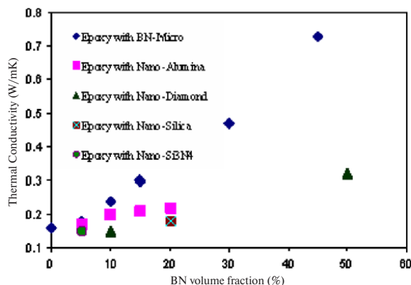
Рис. 3. Теплопроводность эпоксидных композитов, наполненных микро- BN, нано- \text{Al}_2\text{O}_3 , наноалмазами, нано- \text{SiC} и наноаморфными частицами \text{Si}_3\text{N}_4
