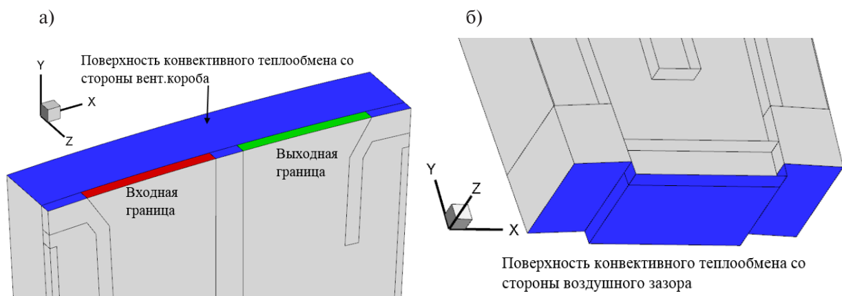
Рис. 4. Граничные условия со стороны вентиляционного короба (а) и воздушного зазора (б)
